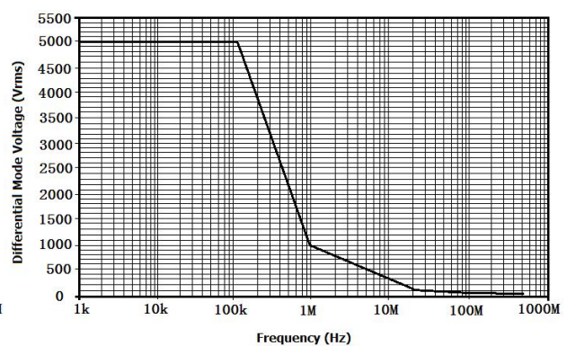
图 4 DPR6700A 最大差模电压 VS 频率
