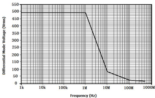
图 1 DPR6070A 最大差模电压 VS 频率
