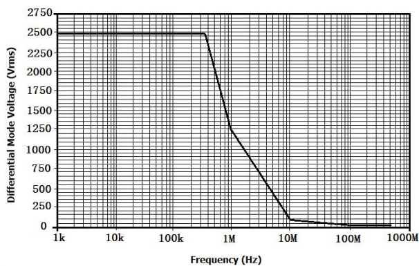
图 3 DPR6350A 最大差模电压 VS 频率
