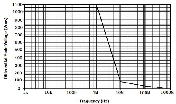
图 2 DPR6150A 最大差模电压 VS 频率
