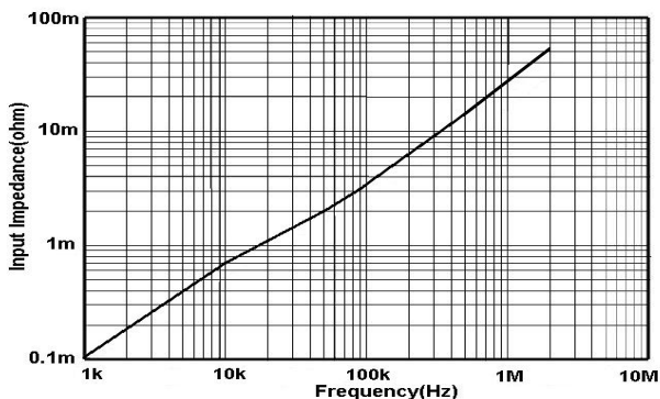
图 3 TCP8102 输入阻抗 VS 频率曲线
