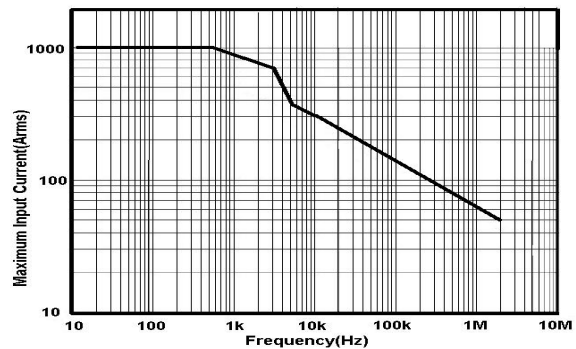
图 2 TCP8102 最大测量电流 VS 频率曲线
