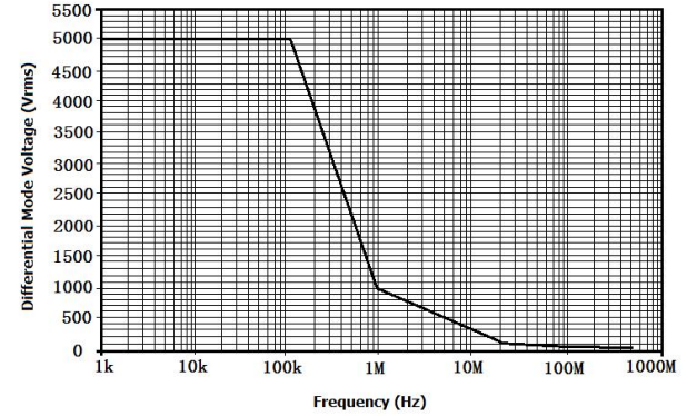
图 4 DPX6700B 最大差模电压 VS 频率
