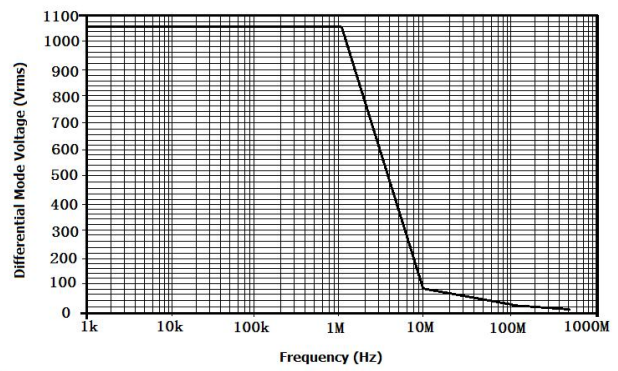
8 图 2 DPX6150B 最大差模电压 VS 频率
