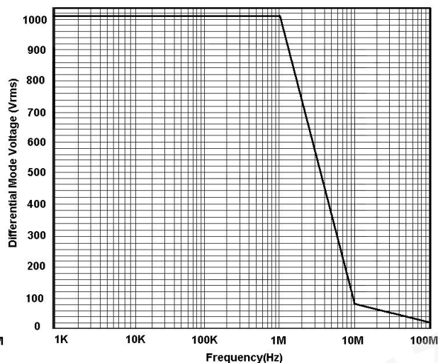
图 2: DP6150 (A/B/D) 最大差模电压 VS 频率
